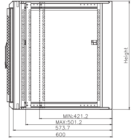
A-A
